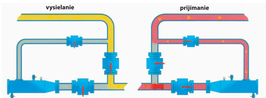
Obr. č. 2 Stará tradičná cesta vkladania a vyberania čistiaceho krtka
